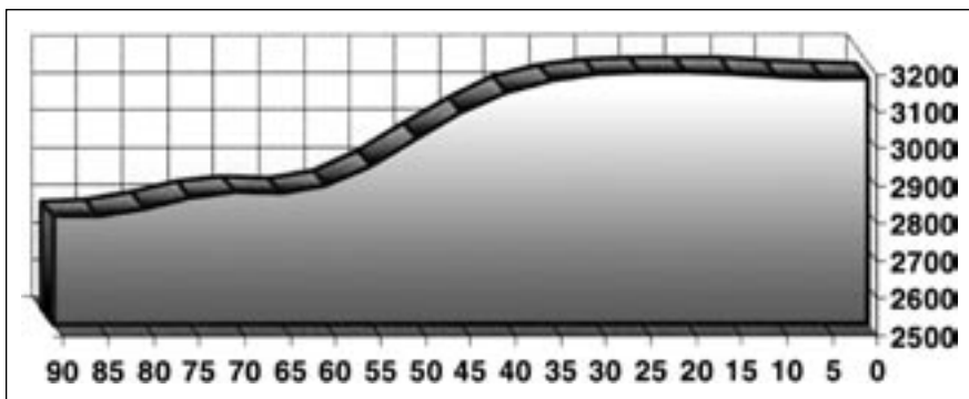
Figura 6. Topografía hemisférica de la superficie de presión de 700 hPa en mdp (1980-2004) (Dattore, B. and Spangler, W., 2005). El gradiente hemisférico de presión es fiel reflejo de las dos masas de aire o fluidos que interaccionan sobre la zona de las latitudes medias.
