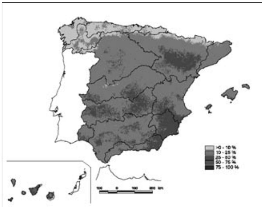
Figura 2. Libro Blanco del Agua. Escenario n° 2. Impacto sobre los recursos hídricos a través de la reducción de la escorrentía. La Región mediterránea podría sufrir una grave reducción de hasta el 50% en sus escorrentías.
